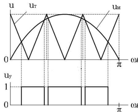
Рис. 1. Діаграми формування імпульсів керування транзисторними ключами АТП
