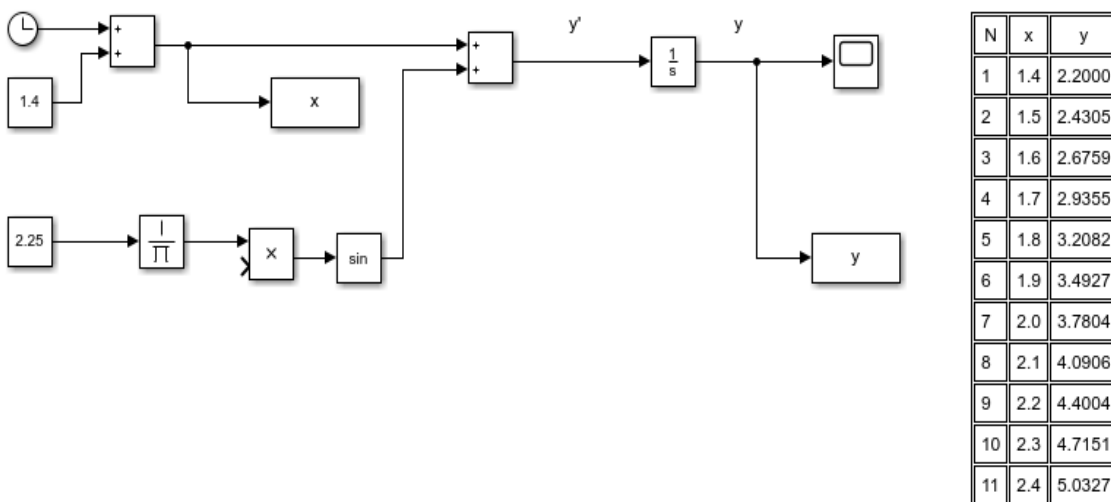
Рис. 1. Структурна схема та результати моделювання ДР (4) засобами Matlab Simulink
