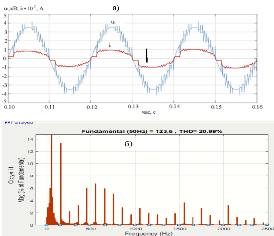
Рис.2. Діаграми електромагнітних процесів при роботі електровоза в режимі тяги на 3-й зоні регулювання : а) осцилограма напруги U_1 і струму i_1 первинної обмотки ТТ, б) спектрограма струму i_1
