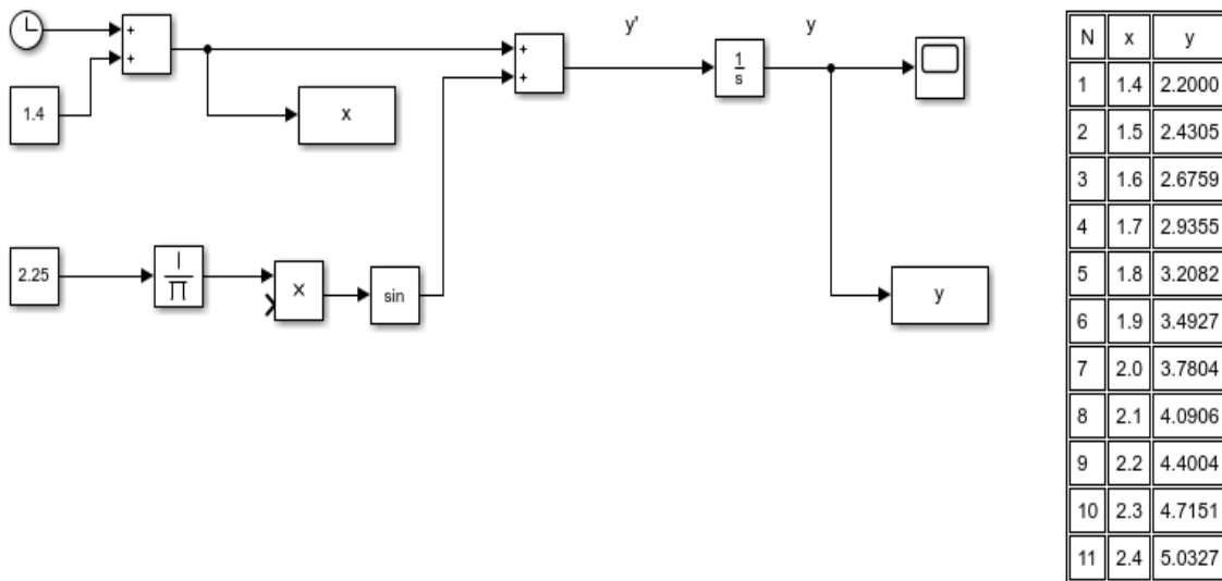
Рис. 2. Структурна схема та результати моделювання ДР (5) засобами Matlab Simulink
