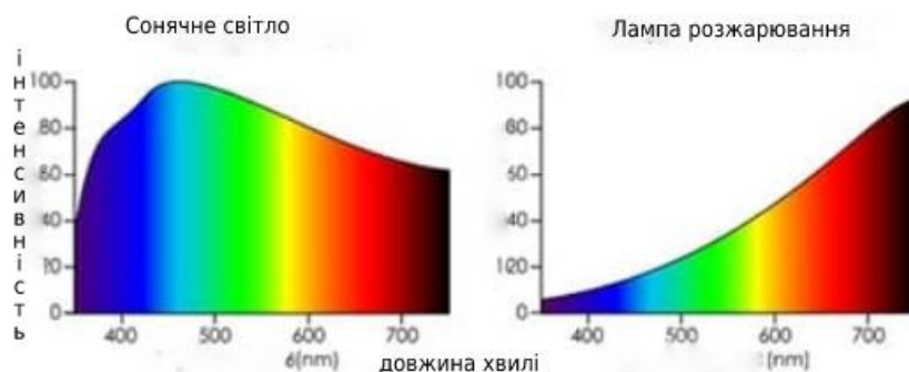
Рис. 2. Порівняння спектрів сонячного світла і лампи розжарювання
