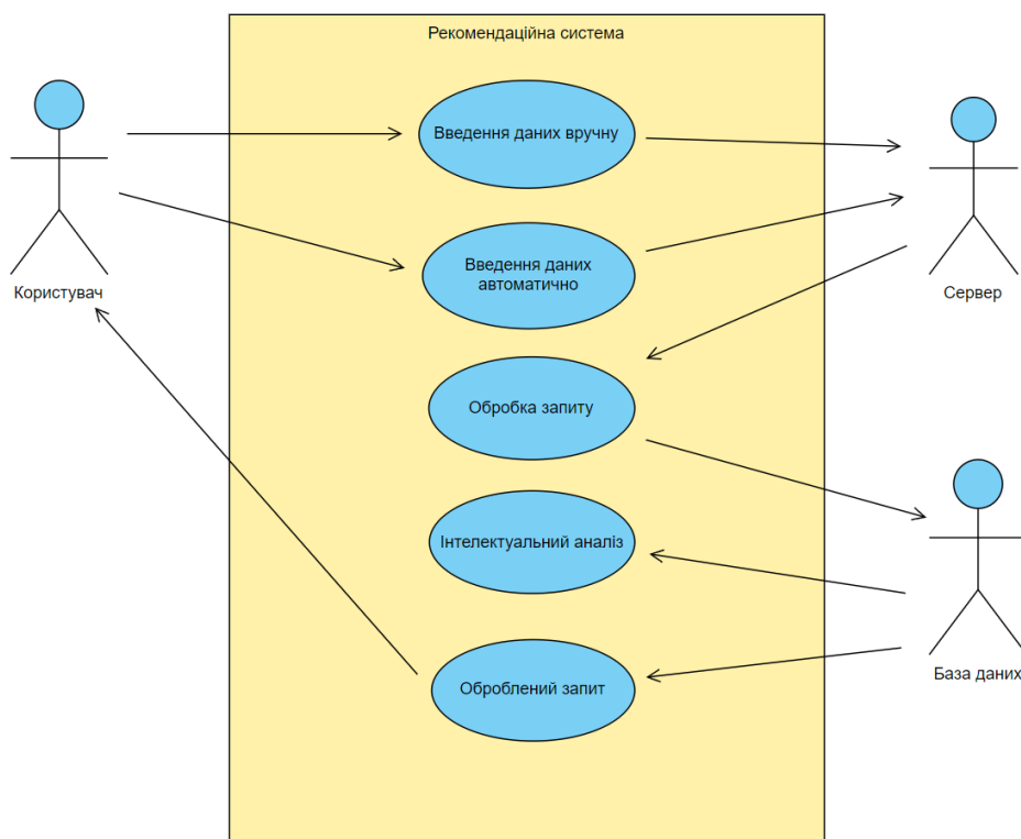
Рис. 1. Діаграма прецендентів системи
