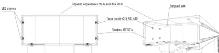
Конструктивний вузол 1
