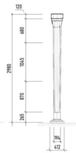
Розріз 1 - 1 M 1: 75
