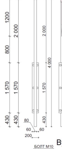
Вид збоку М 1:20
