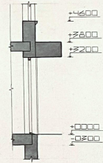
РОЗРІЗ М 1:50
