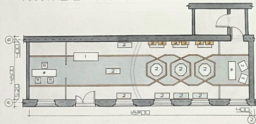
ПЛАН СТЕПІ М 1:25
