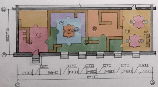
ПЛАН ПІДЛОГИ М1:75
